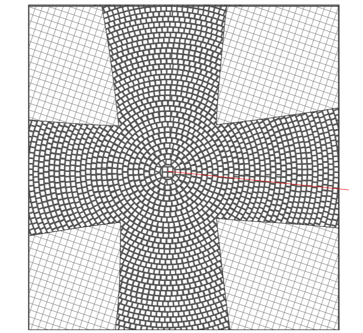
Detalji 2. Ritariaukion ladontamallit 1:100
